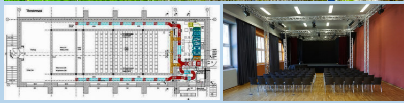
Landesschule Pforta – Einbau einer Lüftungsanlage im historischen Gebäude mit Theatersaal und Bühnenraum Varianten zur Anordnung der Technikräume im vorhandenem Theater, im Bühnen- oder Foyerbereich Bestandsaufnahme, Vorentwurfsplanung
