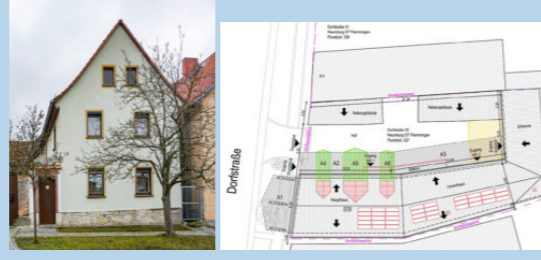
Umbau und Modernisierung denkmalgeschützte Hofanlage, Naumburg (Saale) OT Flemmingen Wohnen für drei Generationen, getrennte Wohneinheiten, historischer Lehm- und Holzbau, Naturstein, moderne Architekturelemente, Pellet-heizung, Nutzung Solaranergie Bestandsaufnahme, Vorentwurfs- und Genehmigungsplanung
