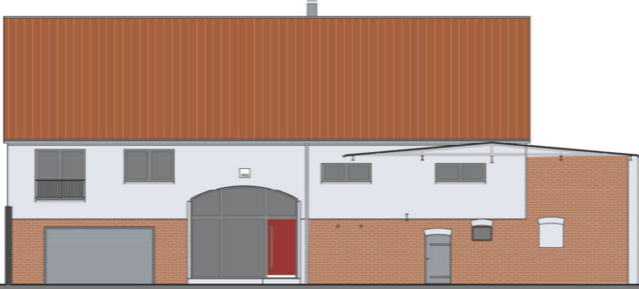
Umbau Scheune zu Wohnhaus, Prititz Bestandsaufnahme, Genehmigungsplanung, Einbau neue Geschossebene, Fassadengestaltung, Pellettheizung, Regenwassernutzung
