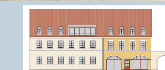
Umbau und Modernisierung Wohn- und Geschäftshaus in Naumburg Bestandsaufnahme und Vorplanung, barrierefreie Wohnungen, Laden und Büros, Einbau Aufzug
