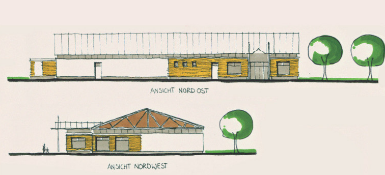
Neubau Verbrauchermarkt Entwurfsplanung
