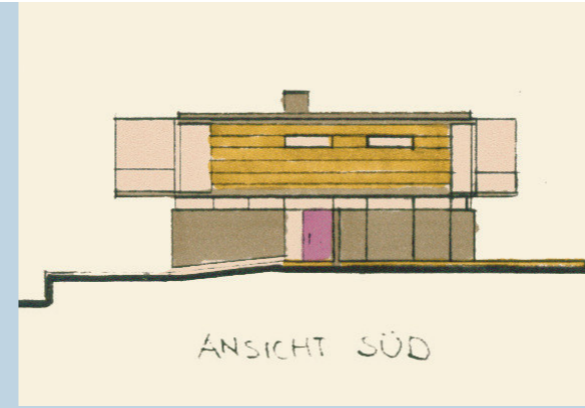
Neubau Zweifamilienhaus Am Georgetor in Naumburg Entwurfsplanung
