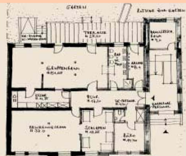
Umbau Stadtvilla zur Kinderkrippe in Naumburg Vorentwurf
