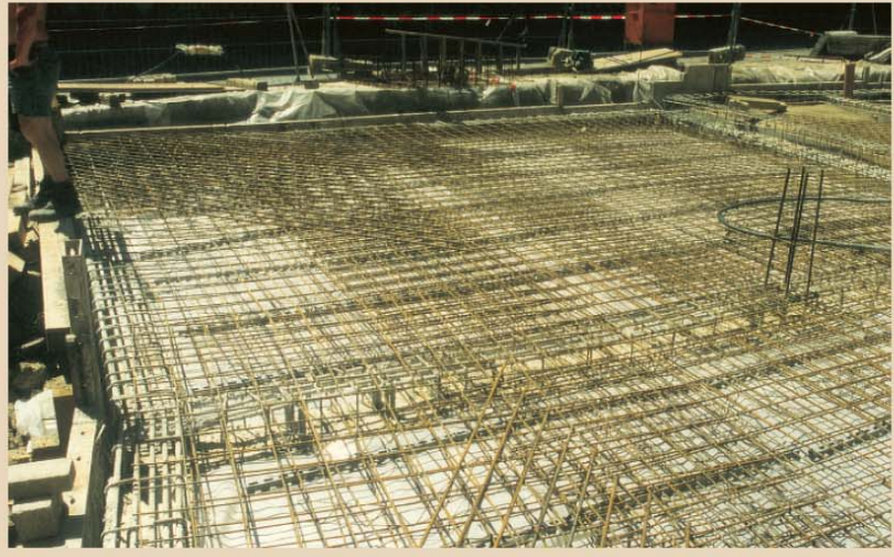
Neubau Wohn- und Geschäftshaus Michaelisstr. 1-2 Bewehrungslage Bodenplatte
